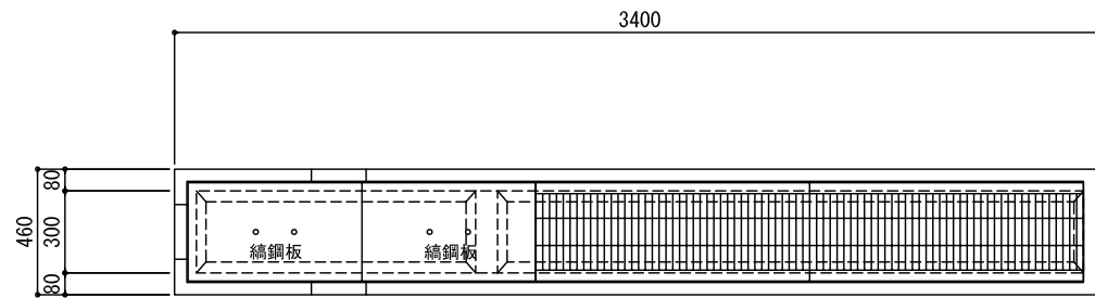
正面図
