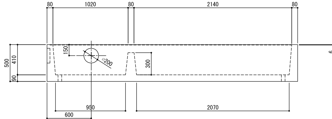
正面図
