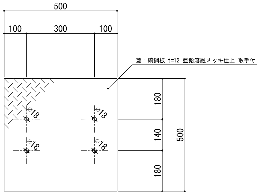
平面図
