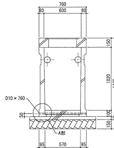
断面図
