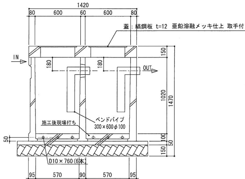
横断面図
